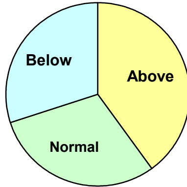
Invercargill Summer Temperatures in La Niña
