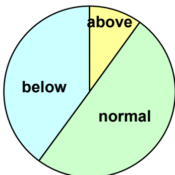
Auckland Summer Temperatures in El Niño
