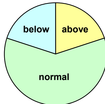
Auckland Summer Temperatures in La Niña
