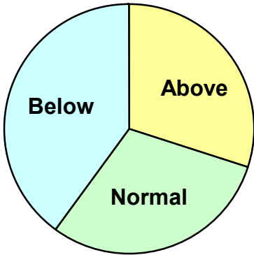
Invercargill Summer Temperatures in El Niño
